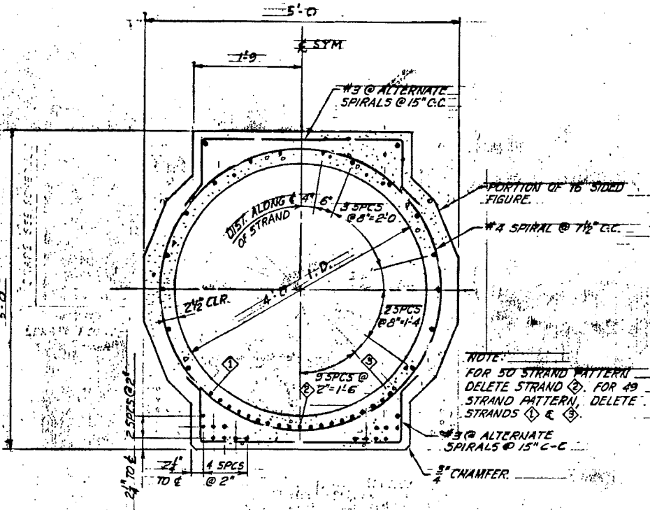
CENTER SECTION SCALE: 1" = 1'-0"
