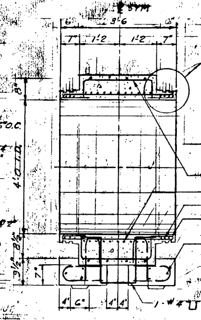
SECTION 4 SCALE: 3/4" = 1'-0"
