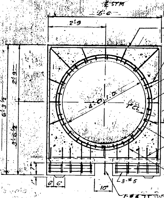
SECTION 3 SCALE: 3/4" = 1'-0"
