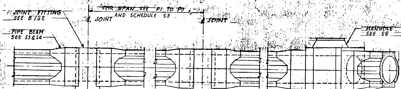
CONDUIT PLAN SCALE: 1/4" = 1'-0"
